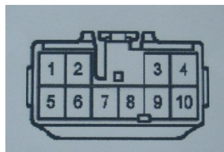
Connettore F45/ F113
